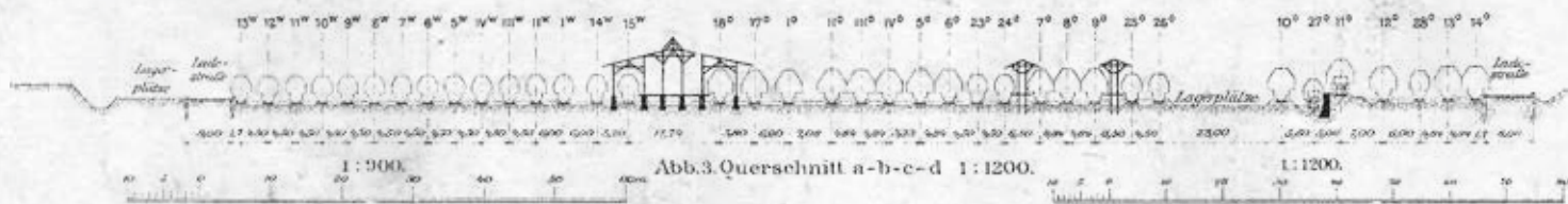
Przekrój peronów
